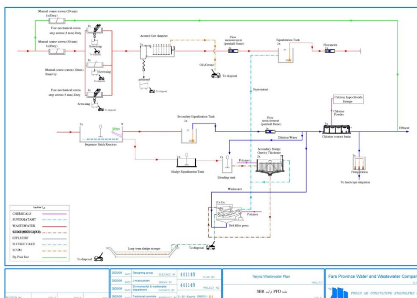
شکل ۳- جنرال پلان طرح احداث تصفیه خانه فاضلاب
